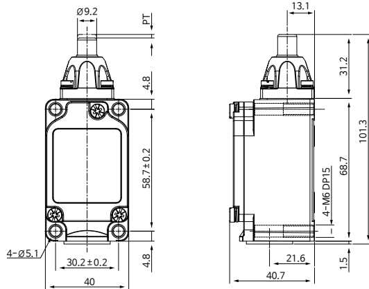
꺾 플러저형 KXL -303
