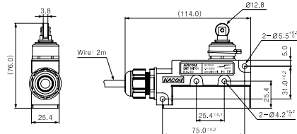
롤러 플런저형 ELN-030
