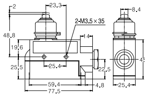
플런저형 E1Z4P1K1
