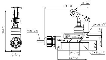
롤러 레버 플런저형 ELN-09
