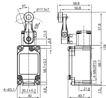
가변 롤러 레버형 KXL -713
