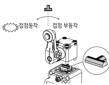
레버 좌측 회전 시에만 접점 동작
