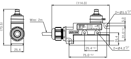
푸쉬 플런저형 ELN-03
