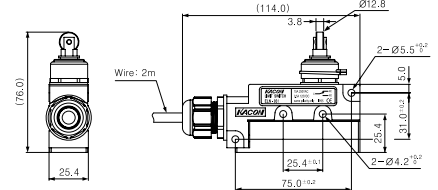
크로스 롤러 플런저형 ELN-031
